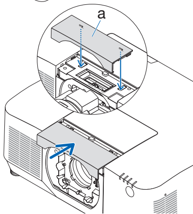
a：鏡頭罩
